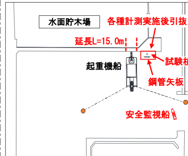
施工平面図
